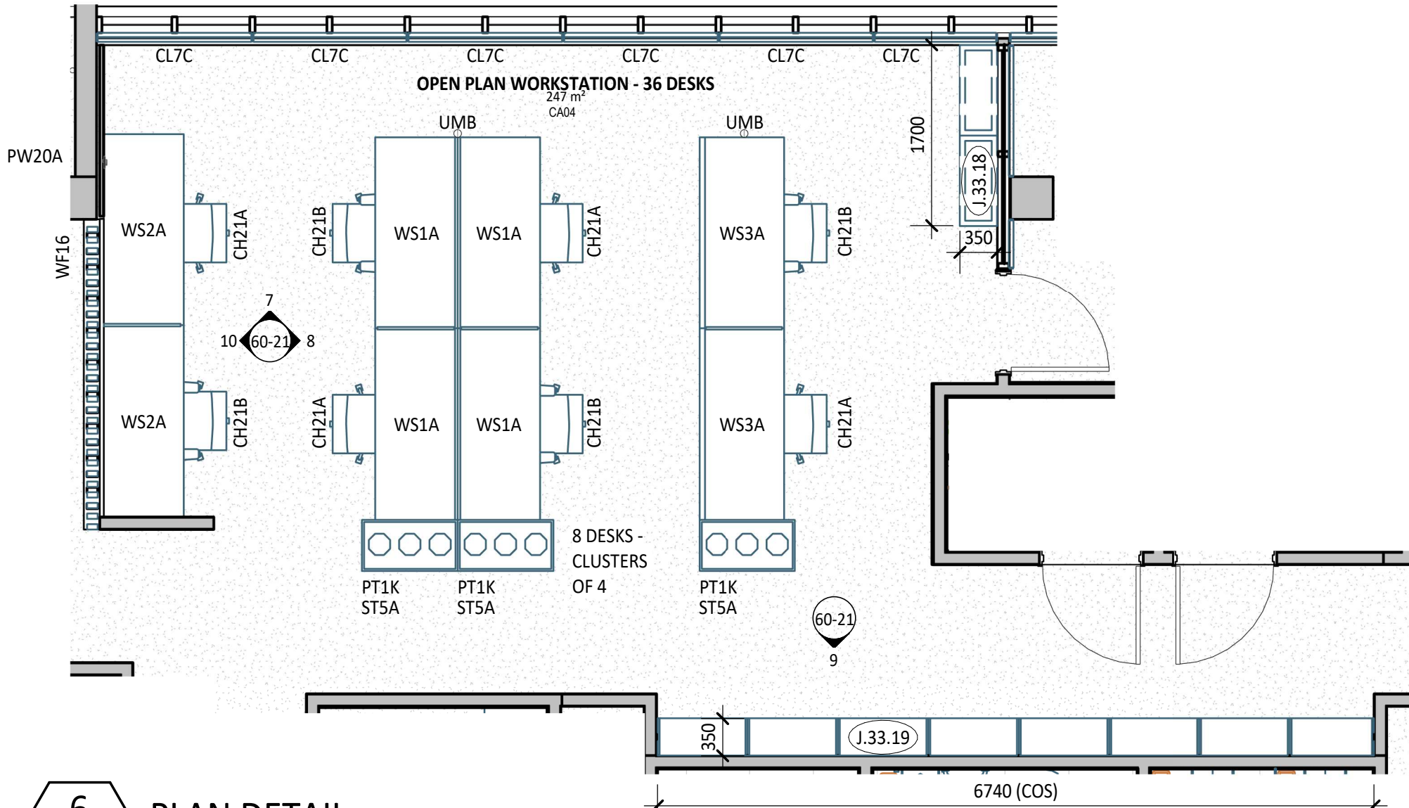
6 PLAN DETAIL 1 : 50
