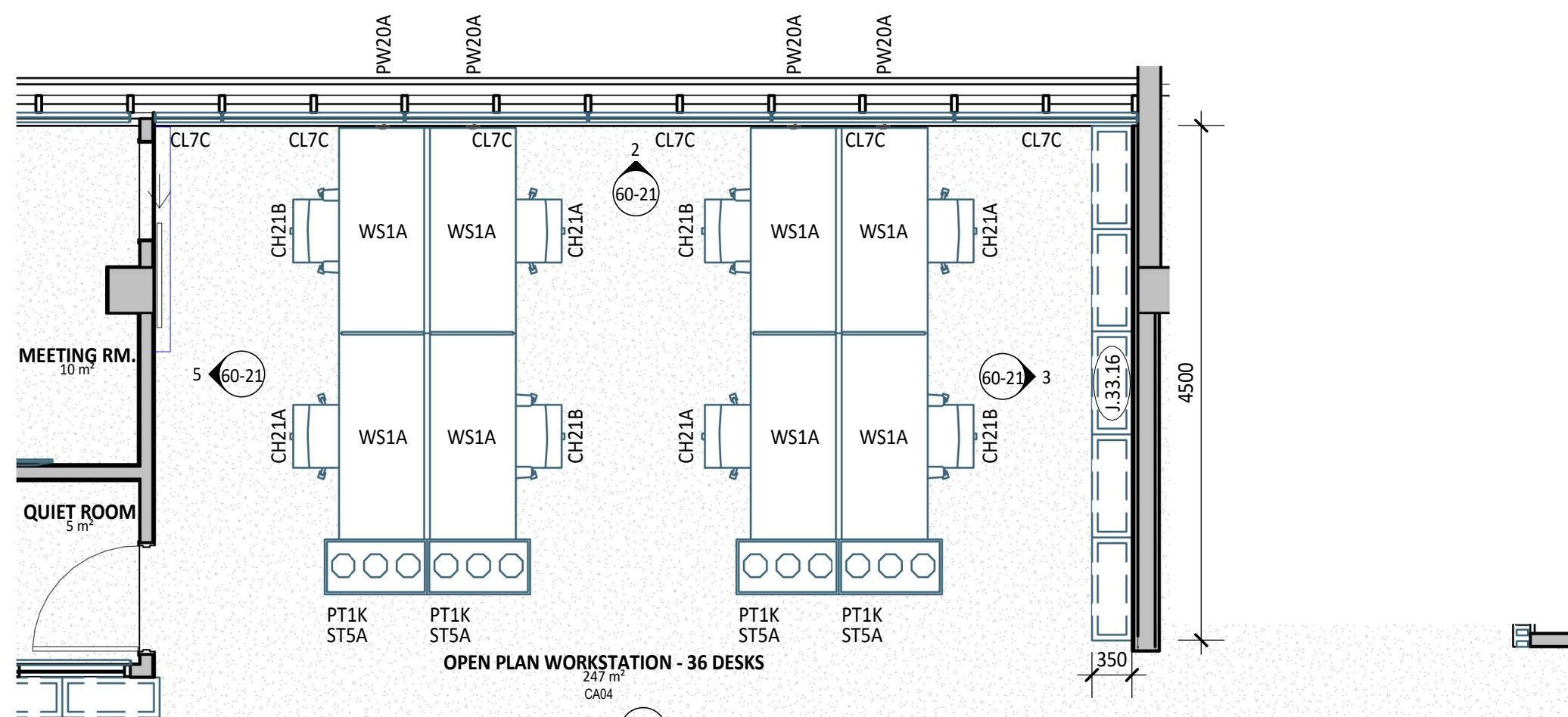
1 PLAN DETAIL 1 : 50
